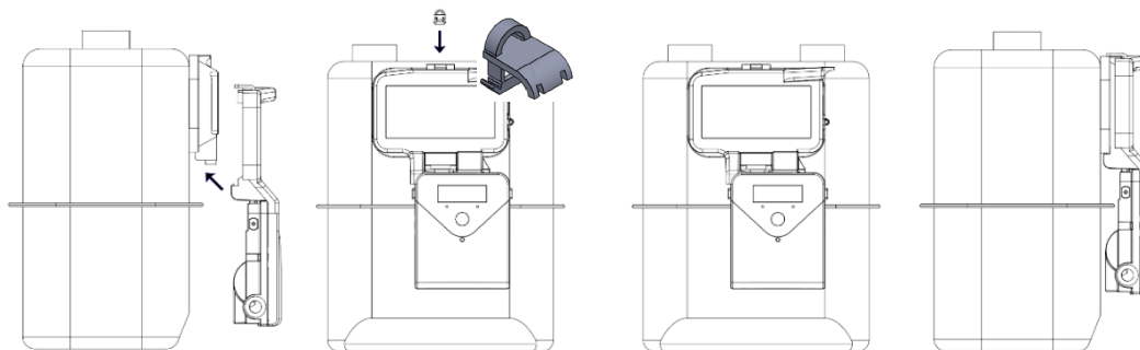
MacR8 montaż do gazomierza ITRON.
