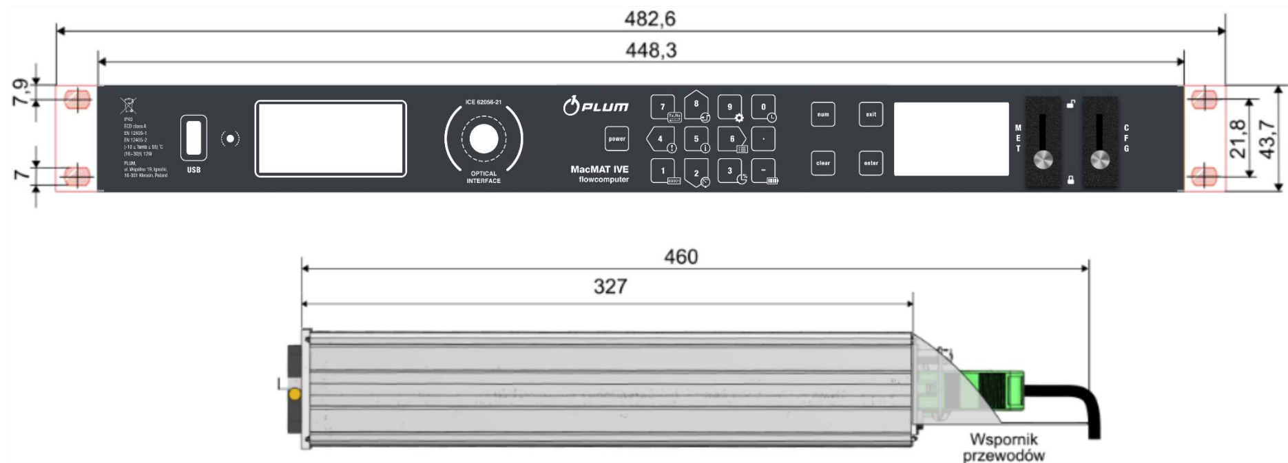
Wymiary i rzut techniczny obudowy przelicznika.
