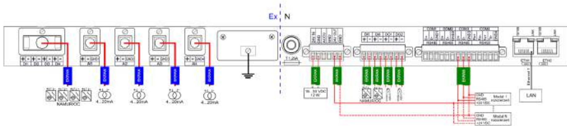
Wyrowadzenia złącz i opis zacisków iskrobezpiecznych i nieiskrobezpiecznych przelicznika.
