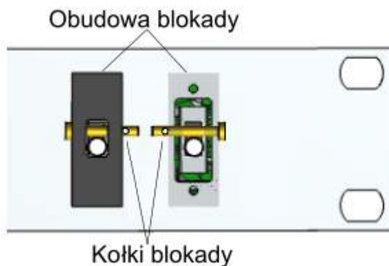
Mechaniczna blokada programowania i metrologiczna przelicznika.
