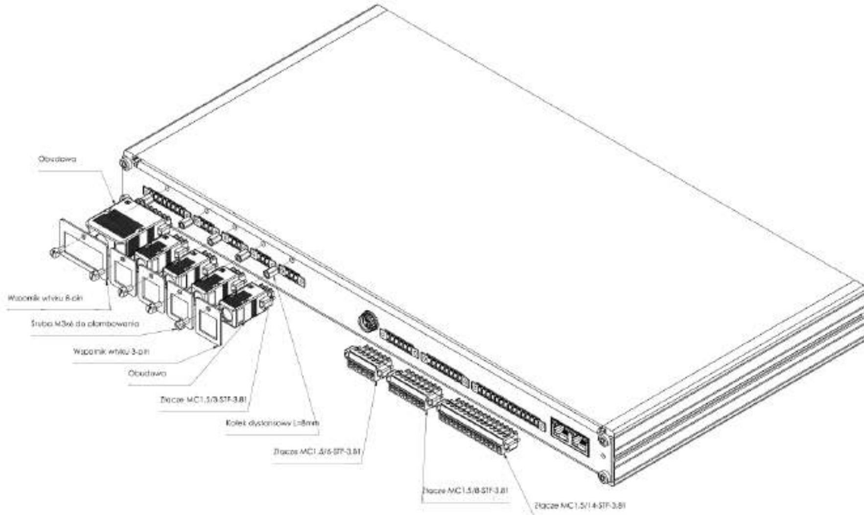
Typy zastosowanych złączy i wtyków do gniazd przelicznika.
