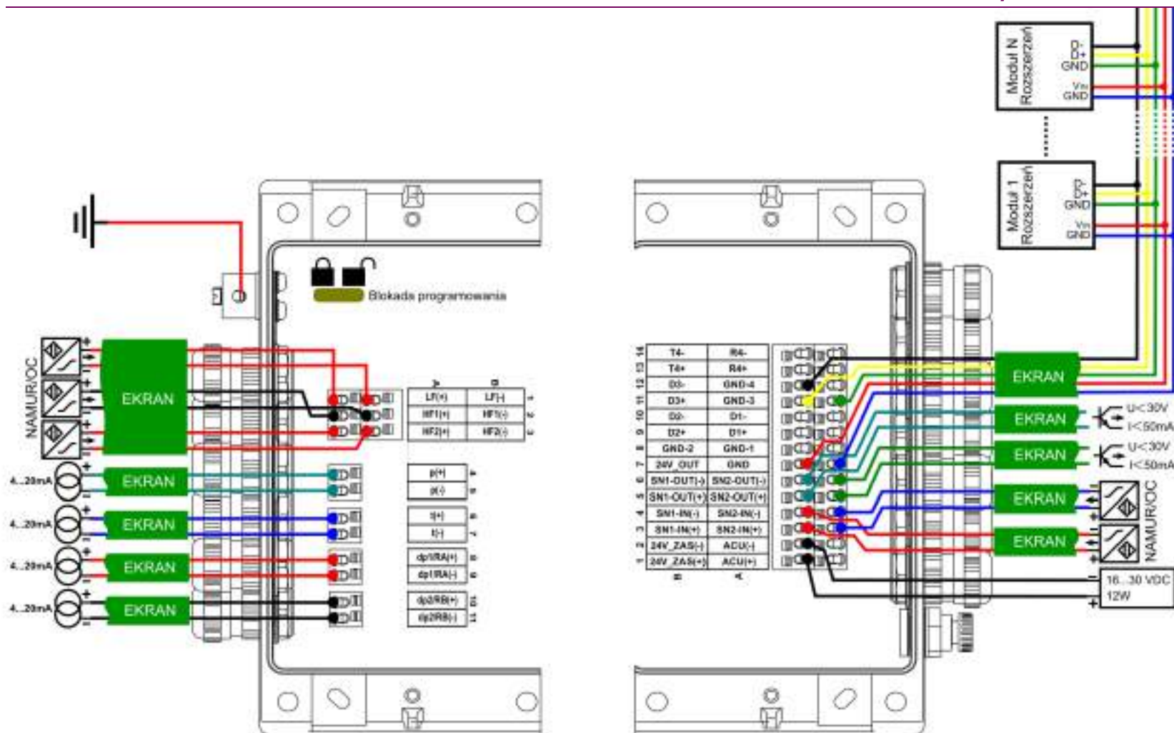
Rys. 1 Schemat połączeń listew zaciskowych przelicznika MacMAT IV w wykonaniu/Nx
