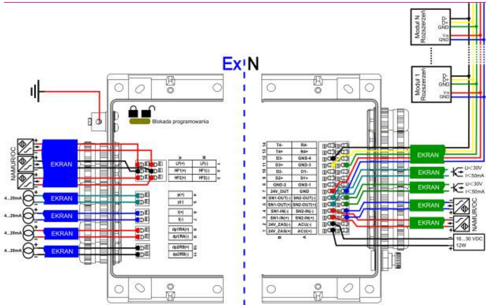
Rys. 2 Schemat połączeń listew zaciskowych przelicznika MacMAT IV w wykonaniu/Ex
