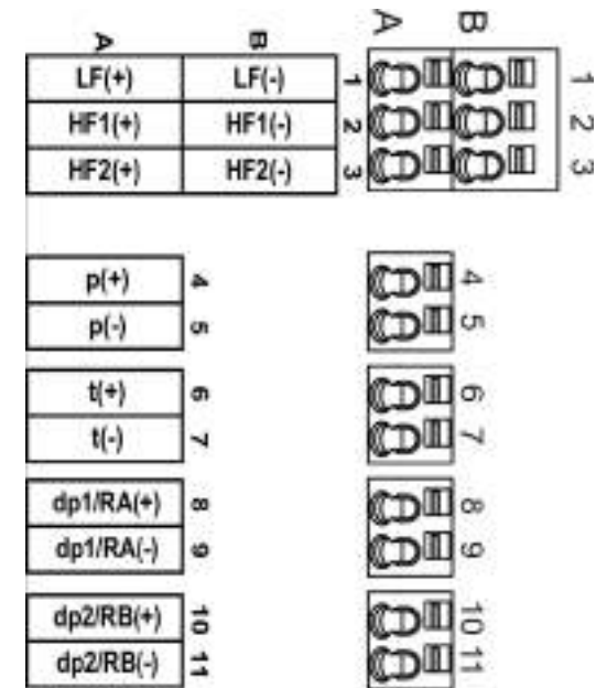
Rys. 10 Zaciski obwodów pomiarowych
