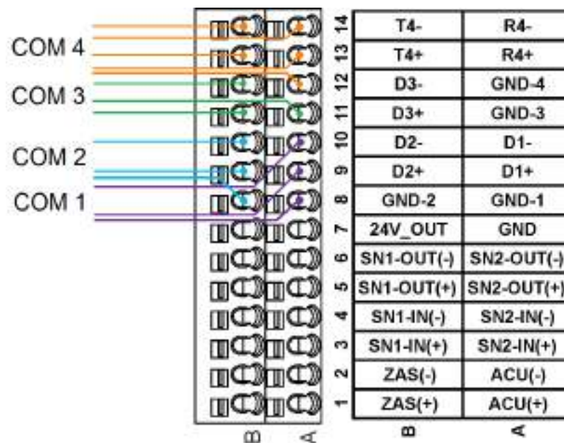
Rys. 12 Zaciski obwodów nieiskrobezpiecznych – połączenie portów transmisji
