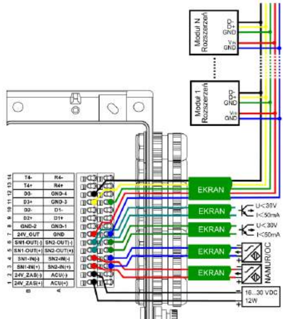
Rys. 11 Sposób podłączenia obwodów sygnalizacyjnych
