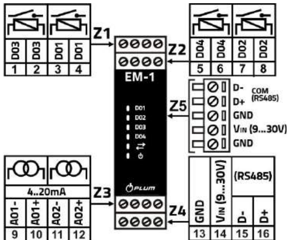
Rys. 33 Rozmieszczenie wejść/wyjść modułu EM-1
