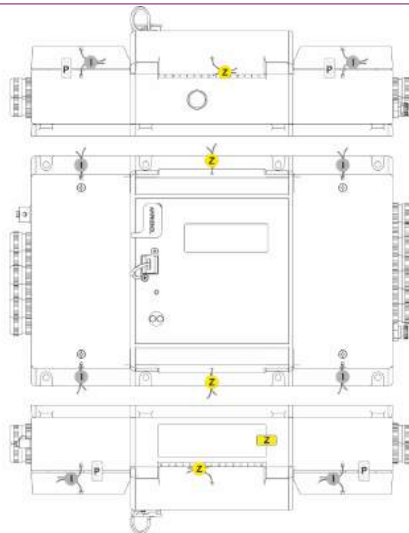
Rys. 5 Schemat przedstawiający rozmieszczenie plomb na przeliczniku
