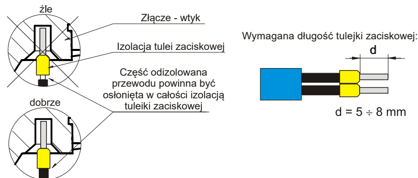
Rys. 8 Zakładanie końcówek tulejkowych
