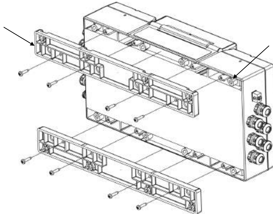
Rys. 3 Sposób montażu przelicznika przy pomocy specjalnych uchwytów
