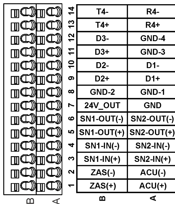
Rys. 13 Zaciski obwodów sygnalizacyjnych
