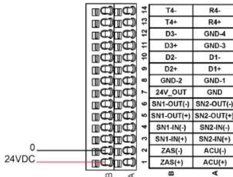
Rys. 9 Zaciski obwodów nieiskrobezpiecznych
