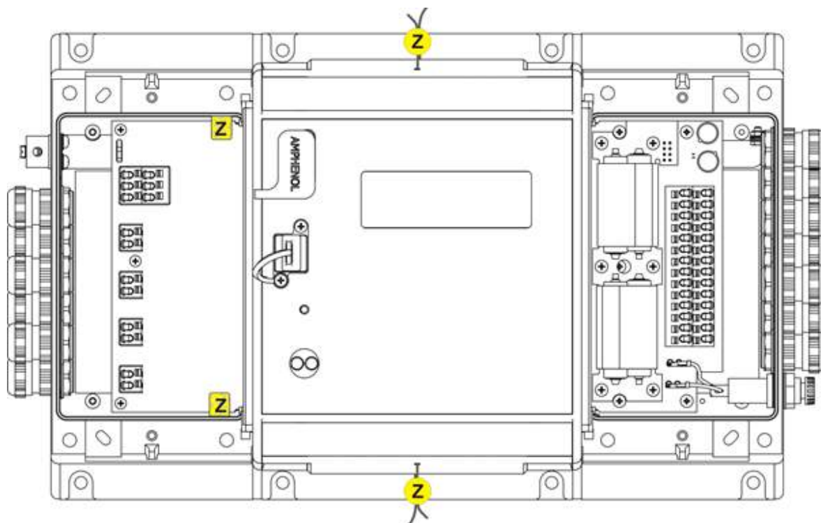
Rys. 6 Schemat plombowania wewnętrznego
