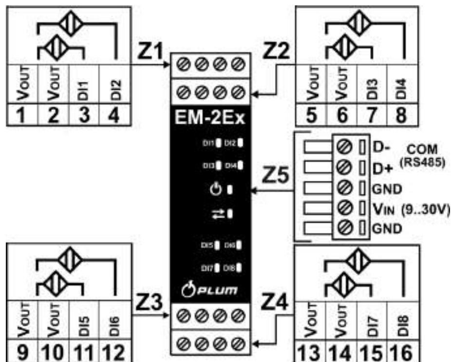
Rys. 34 Rozmieszczenie wejść modułu sygnalizacji
